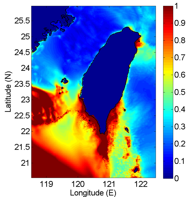
圖3-5馬尼拉海溝編號27號子斷層若發生規模8.5地震的海嘯模擬圖
