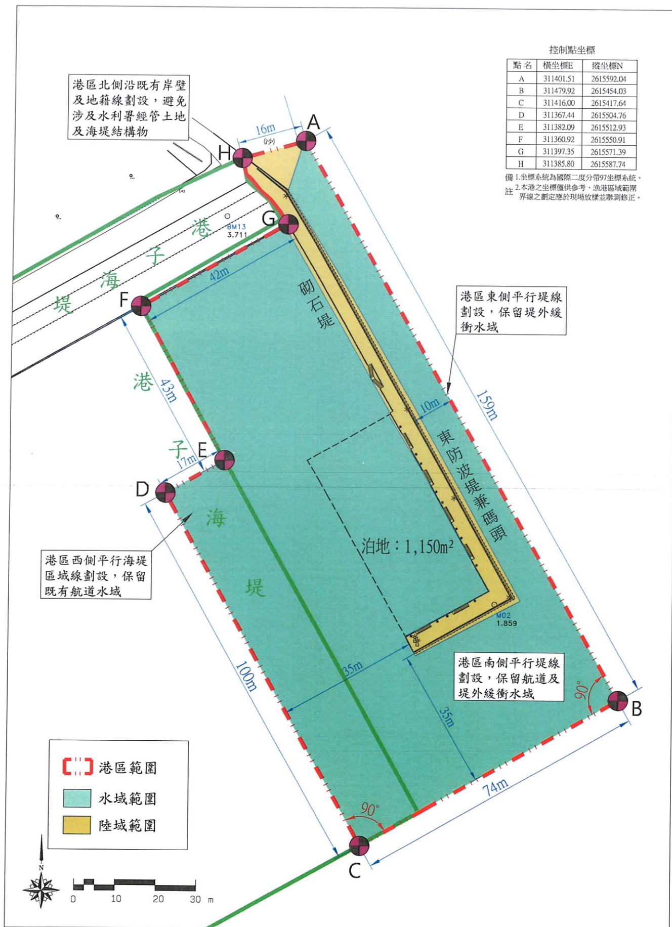
圖3-1 鎮海漁港區域平面圖
