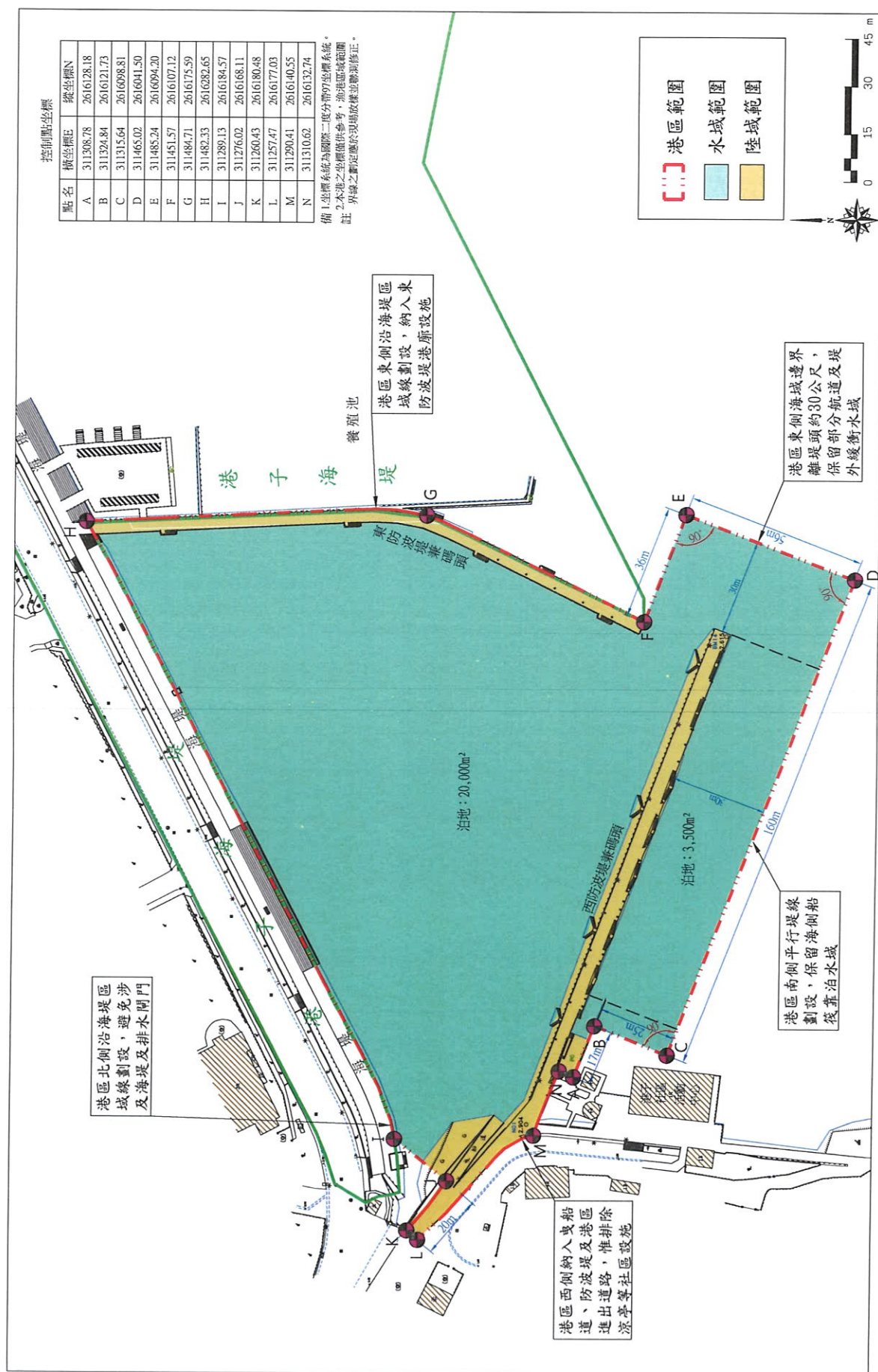
圖3-1 港子漁港區域平面圖
