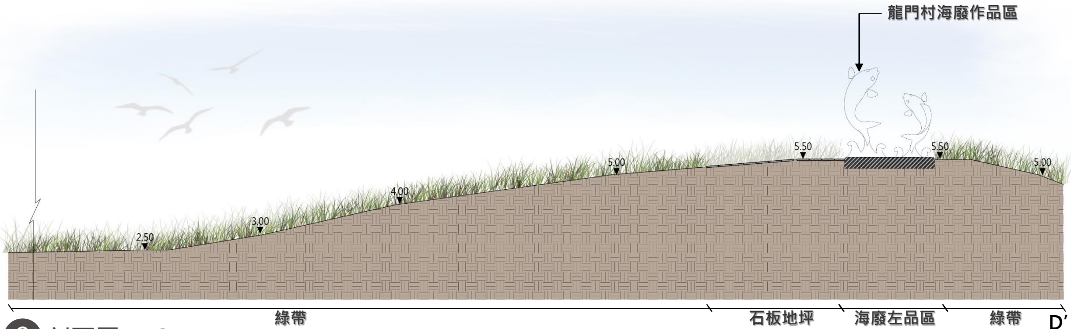
2 剖面圖 D-2
