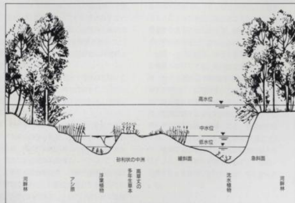
自然に近い流水域の標準断面図
