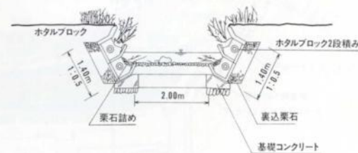
◆ ホタル水路断面図
