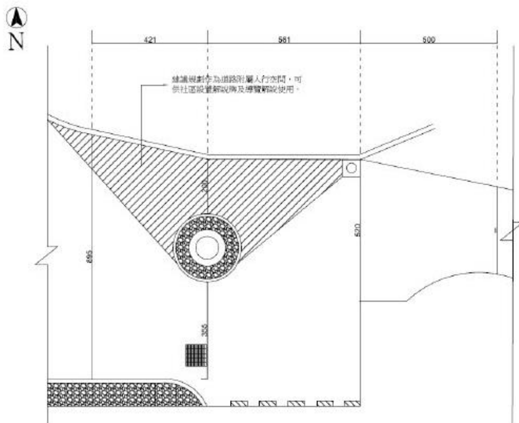
道路附屬人行空間測繪圖
